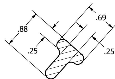
SECTION D-D SCALE 1 : 1
