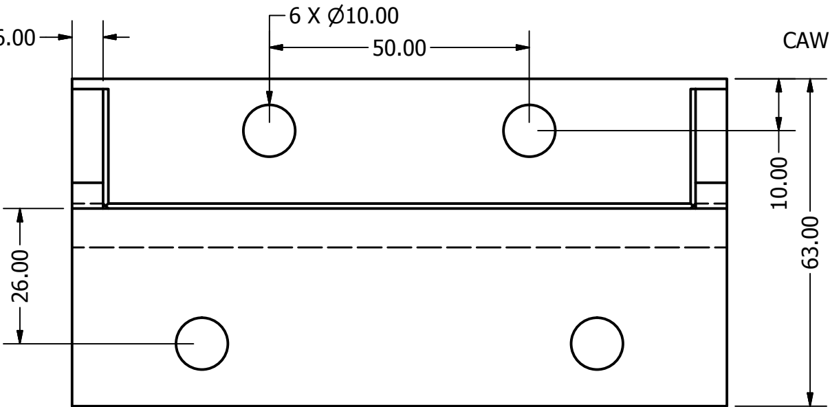
VIEW1 SCALE 1 : 1
