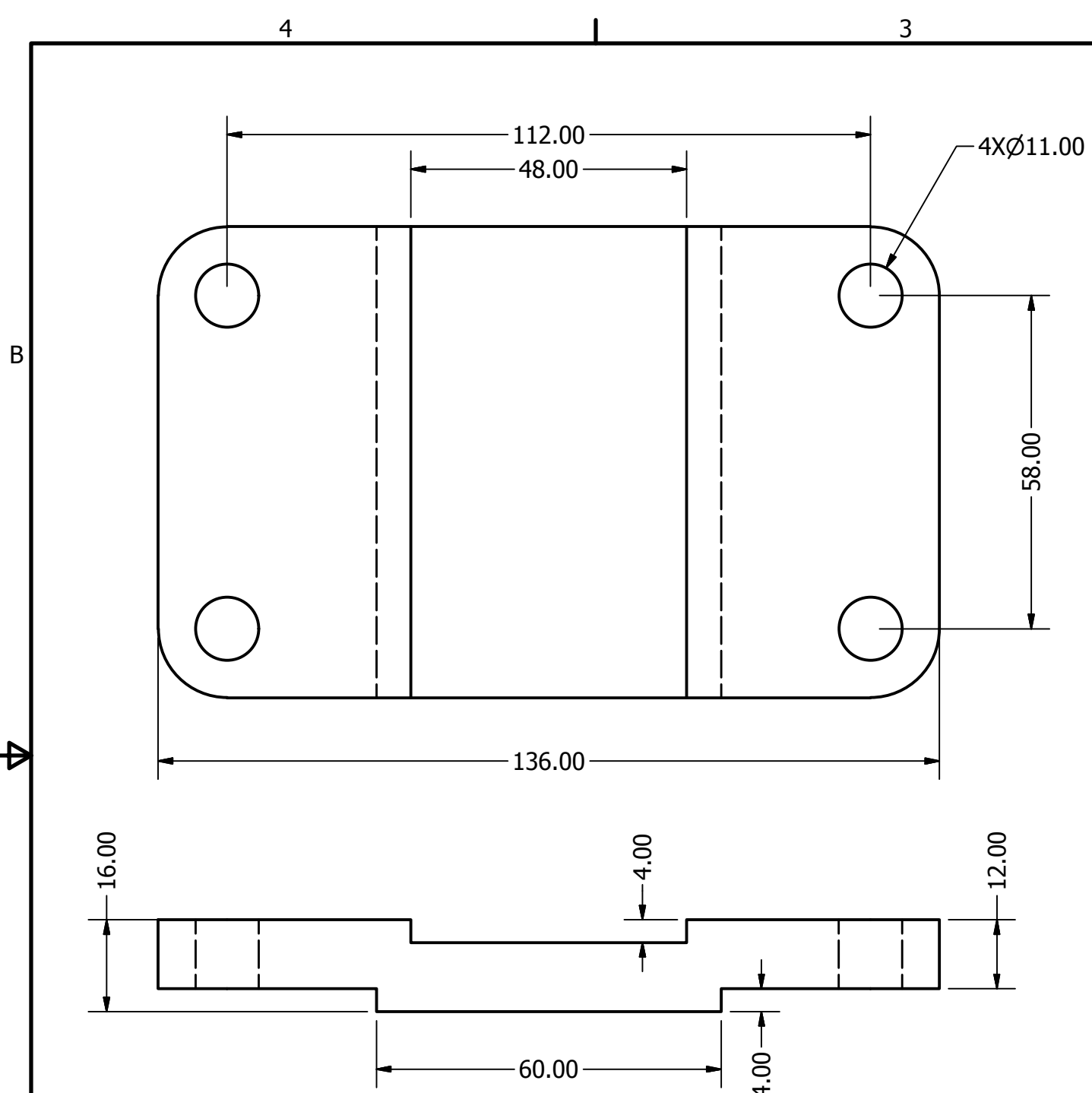
TOP PLATE SCALE 1 : 1
