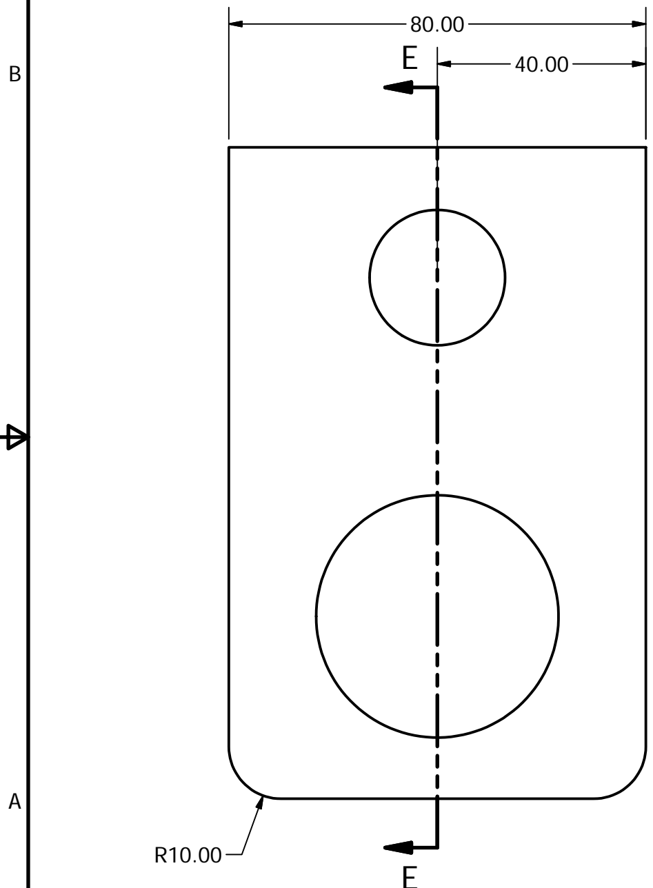
PT4 HANGER SCALE 1 : 1
