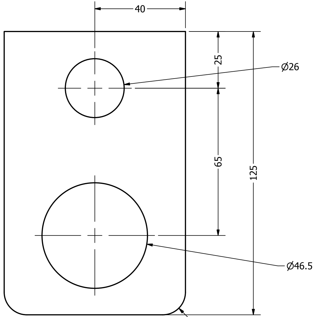
HOOK SCALE 1 : 1
