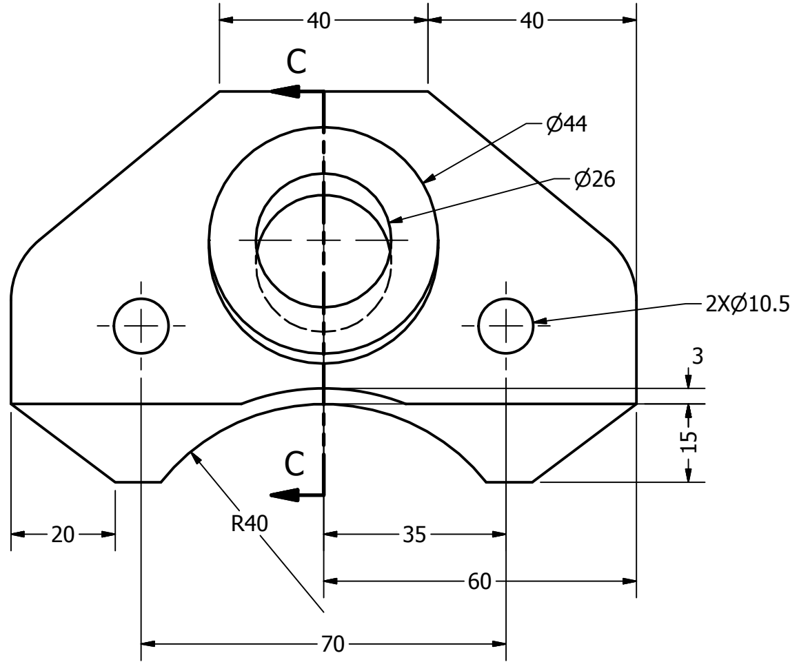
GUIDE SCALE 1 : 1
