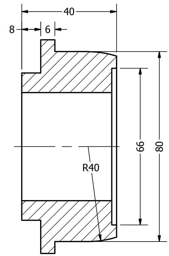
SECTION D-D SCALE 1 : 1
